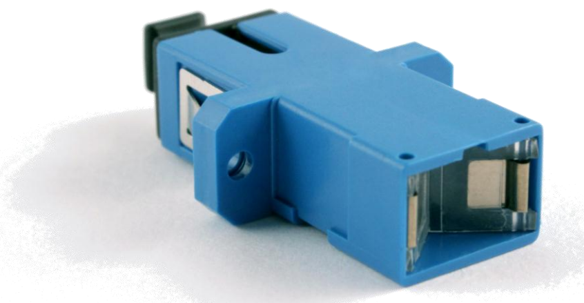
Réf: 48SMTSCSISS Traversée SC/SC simplex auto shuttered, bleue Pour OS1/OS2 et G 657
