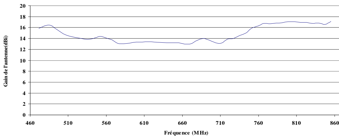
Gain (dBi) en fonction de la Fréquence (MHz)
